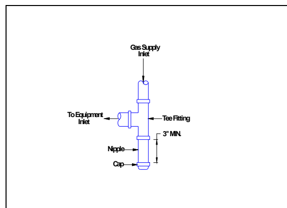
SEDIMENT TRAP
