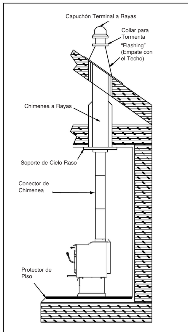
Figura 5.2 Chimenea Prefabricada Interior
