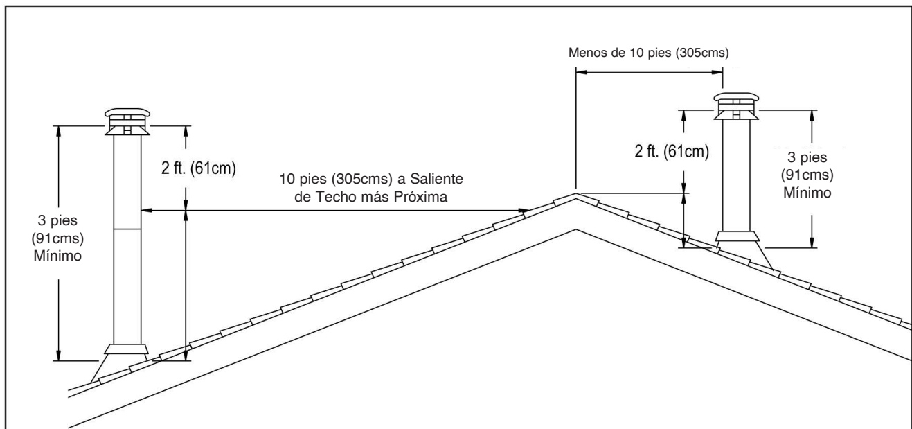
Techo Inclinado
